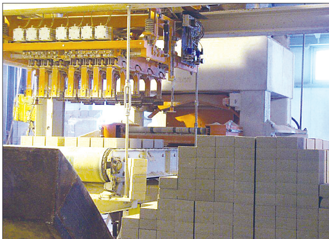
Высокопроизводительное оборудование немецкой компании W+K обеспечивает выпуск кирпича отличного качества
