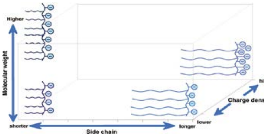
Рис. 1. Разнообразие типов PCE марок MELFLUX и компаундов на их основе MAPF
