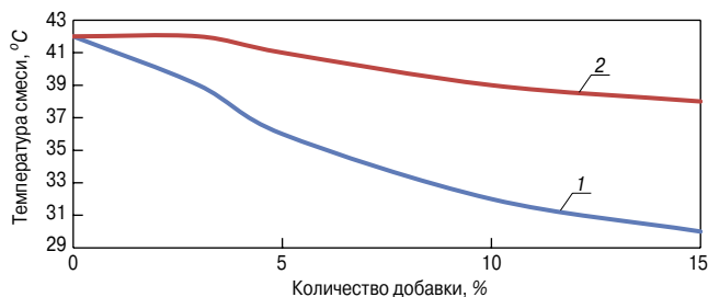
Рис. 9. Влияние комплексной добавки на температуру смеси: 1 – Тсм К-1; 2 – Тсм К-2
