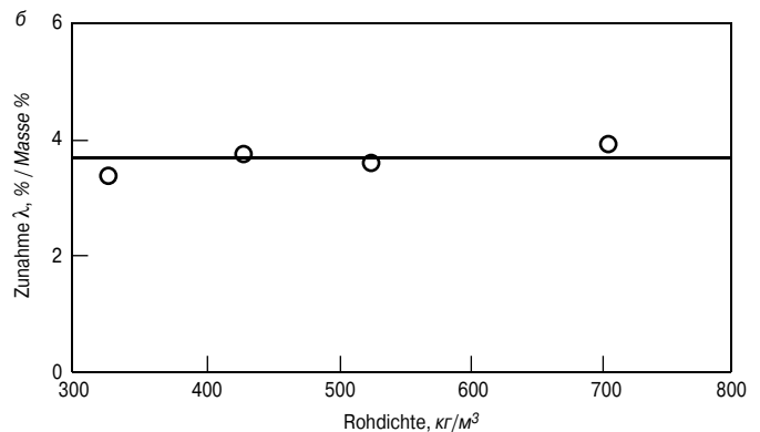
Рис. 2. Зависимость КТК газобетона от плотности: а – по результатам экспериментов; б – из [4]
