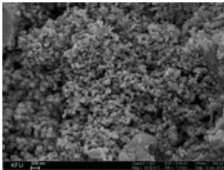
Рис. 3. Вид структуры полимерцементной композиции (П/Ц=0,5) в электронном микроскопе
