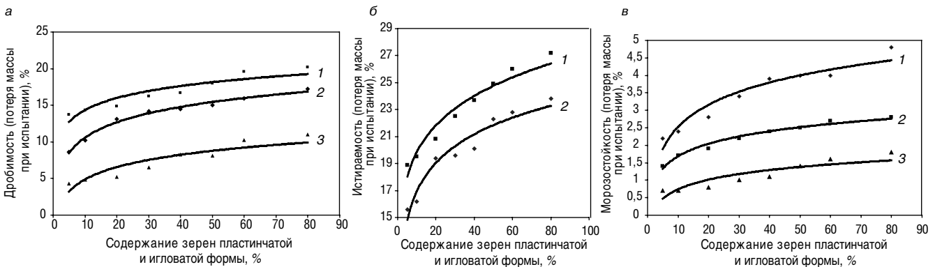
Рис. 1. Влияние содержания зерен пластинчатой и игловатой формы на дробимость (а), истираемость (б) и морозостойкость (в) щебня фракции 10–20 мм из разновидностей гранита 1–3: 1 – гнейсогранит; 2 – микролин-плагиоклазовый гранит; 3 – плагиогранит
