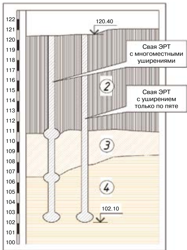
Рис. 1. Инженерно-геологический разрез испытательного полигона и свай, выполненных по электроразрядной технологии, с многоместными уширениями (слева) и только с уширением пятой (справа); вертикальная ось – высотные отметки, м
