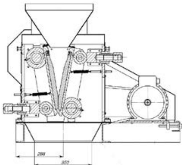
Рис. 3. Схема дробилки 2ЩДС 100×200
