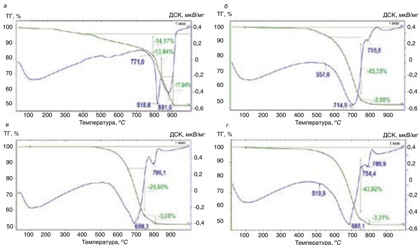
Рис. 2. Дериватогаммы усредненной пробы магнезита 3-го и 4-го сортов Саткинского месторождения фракции: а – ≥ 40 мм; б – 20–40 мм; в – 10–20 мм; г – 10–0 мм.
