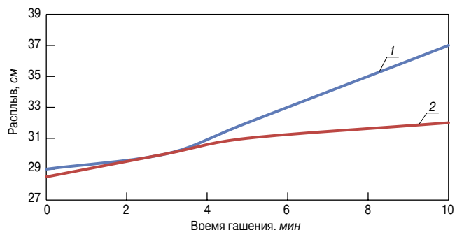
Рис. 8. Влияние комплексной добавки на подвижность смеси: 1 – К-1; 2 – К-2
