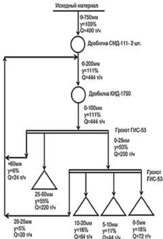
Рис. 2. Технологическая схема производства кубовидного щебня на предприятии «Карат»
