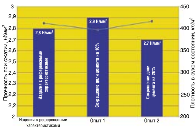
Рис. 6. Результаты лабораторных опытов. Изделие с референсными характеристиками получено без активации и без сокращения количества цемента. Опыты 1 и 2 позволили сократить количество цемента и активацию
