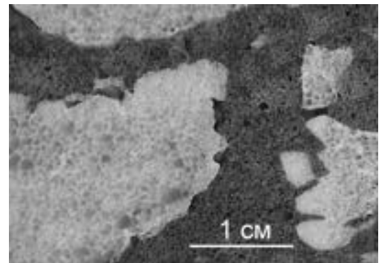
Рис. 2. Фотография среза композиционного материала из белого (окисленного) пеностеклокристаллического щебня на связке из черного (восстановленного) пеностеклокристаллического материала
