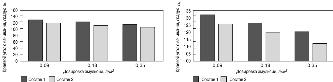
Рис. 7. Влияние дозировки используемой гидрофобной эмульсии на значение КУ смачивания в зависимости от состава цементно-песчаной матрицы: а – с микрокремнеземом; б – с метакеолином
