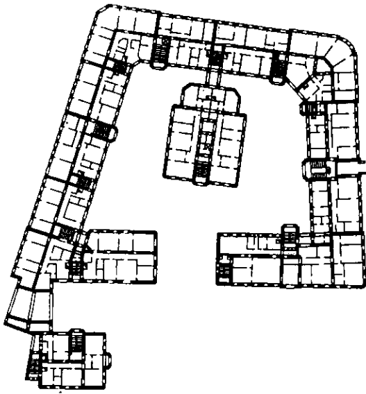
План типового этажа доходного дома Строгановского училища в Москве. Архитектор Ф.Шехтель, 1904 г.
